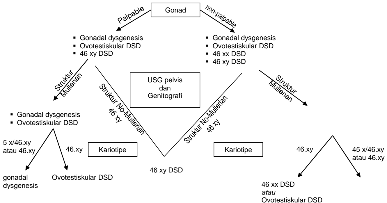
Gambar 4. Algoritme DSD
